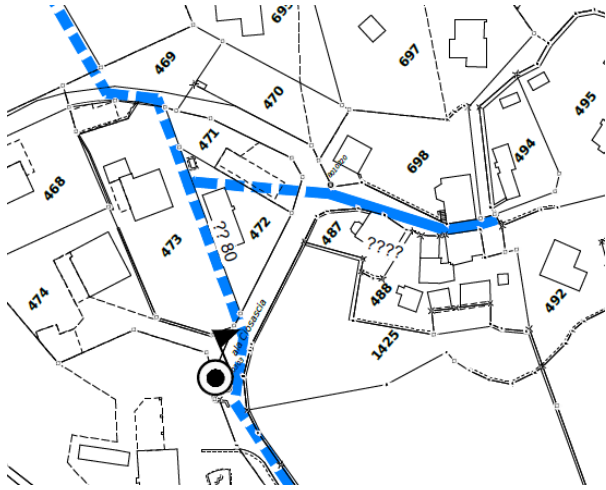
Situazione esistente Nuovo tratto di condotta AP, lunghezza circa 145 ml.
